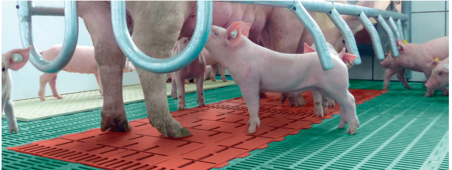
Abb.: Mix-System mit Ferkelnest-Vergrößerungen in Bewegungs-Abferkelbuchten
