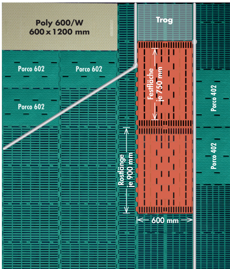
Abb.: Mix-System mit Ferkelnest-Vergrößerungen in Bewegungs-Abferkelbuchten
